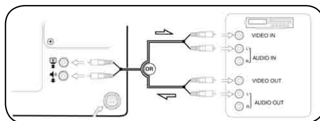
Копирование и/или отображение видеосигнала между внешним видеоустройством и приборной коробкой цветного видеоприбора
