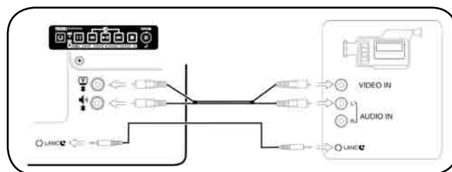
Управление внешним видеомagnetofоном с приборной коробки цветного видеоприбора
