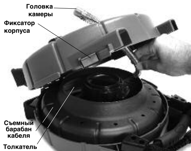
Рис. 3. Внутри корпуса
