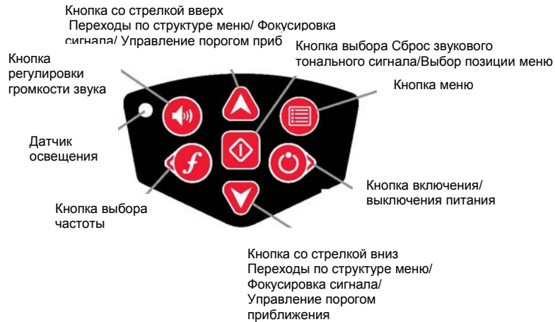
Рис. 5. Кнопочный пульт.
