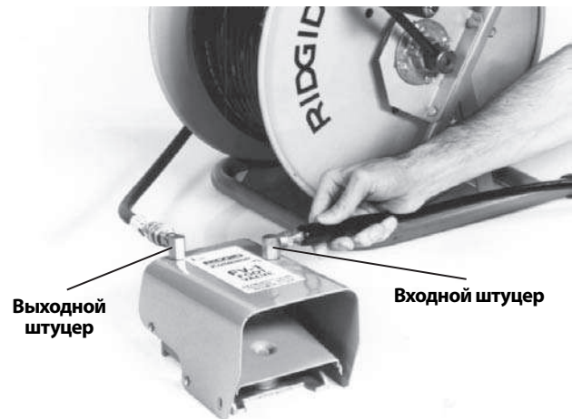
Рис. 11 – Подключение педального клапана
